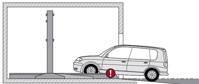
Max. 14% gradient
